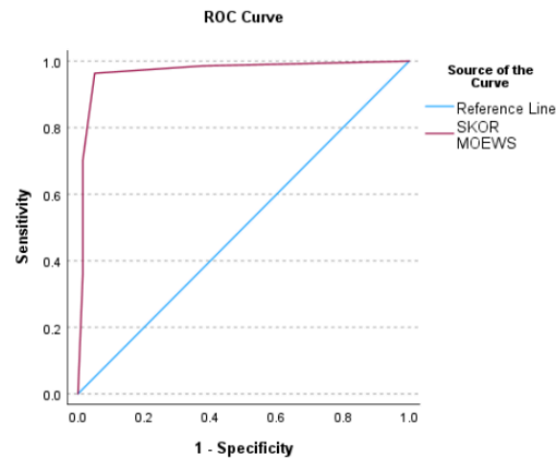
Gambar 1. Kurva ROC
