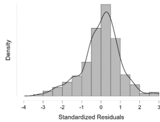
Gambar 1. Uji Normalitas
