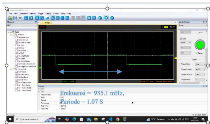
Gambar 11. Pengukuran Osilasi konverter buck sinkron.
