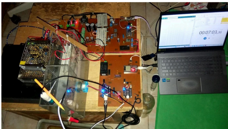
Gambar 14. Pengujian Keseluruhan System
