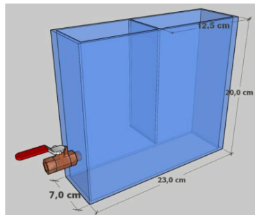
Gambar 3. Desain Reaktor Jar test
