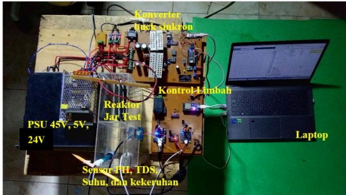
Gambar 10. Realisasi alat.
