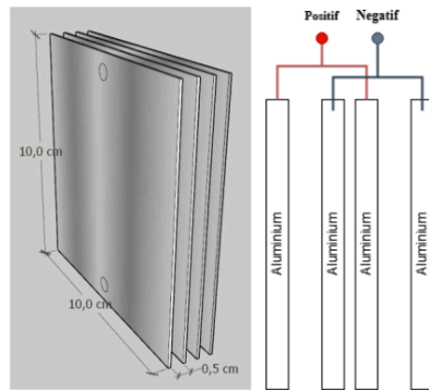
Gambar 4. Desain dan wiring elemen elektrokoagulasi
