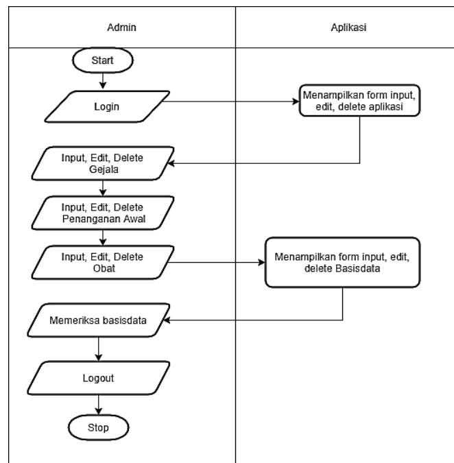
Gambar 5. Diagram aktivitas admin
