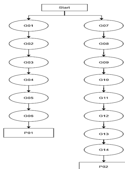
Gambar 7. Pohon keputusan
