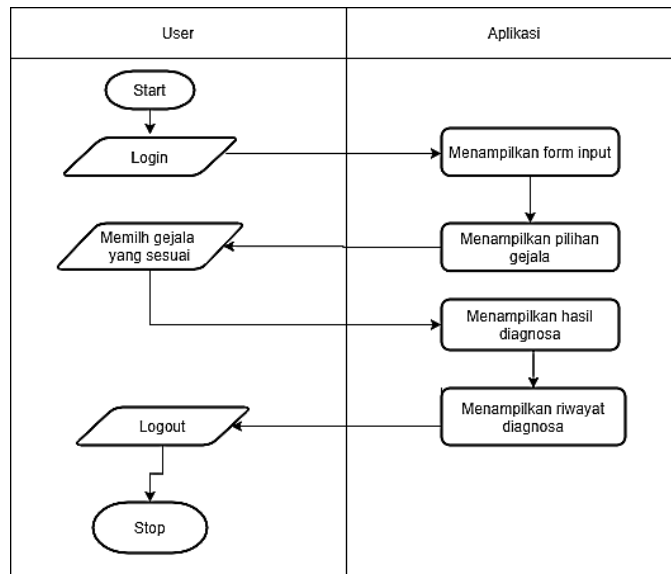
Gambar 4. Diagram aktivitas user
