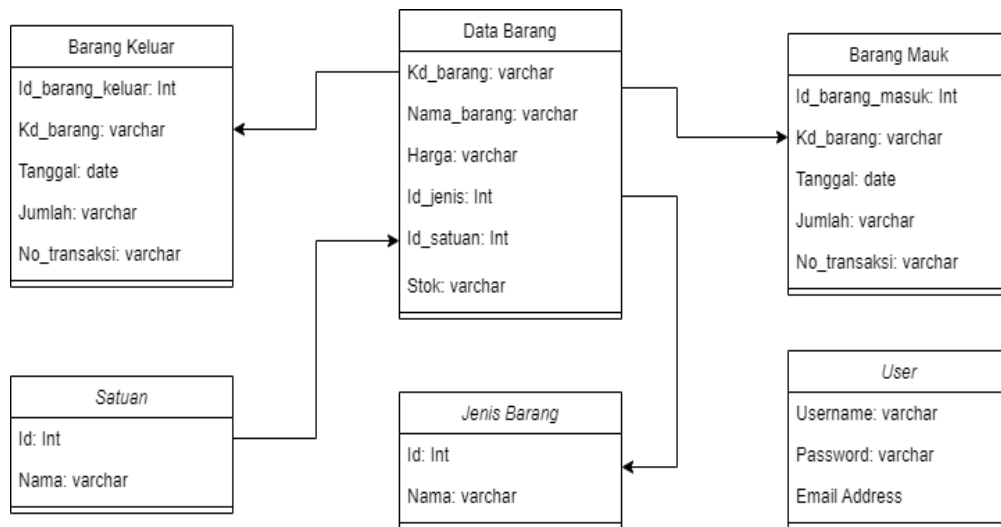
Gambar 4. Relasi Tabel
