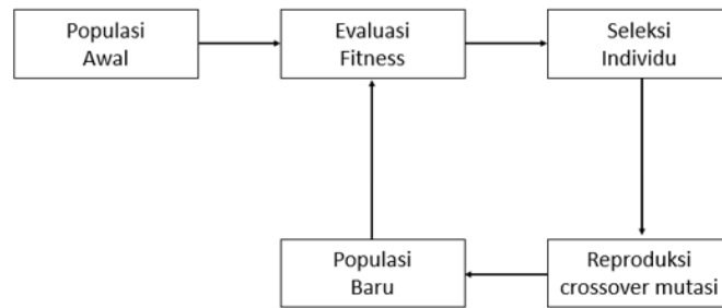
Gambar 2. Algoritma Genetika [31]
