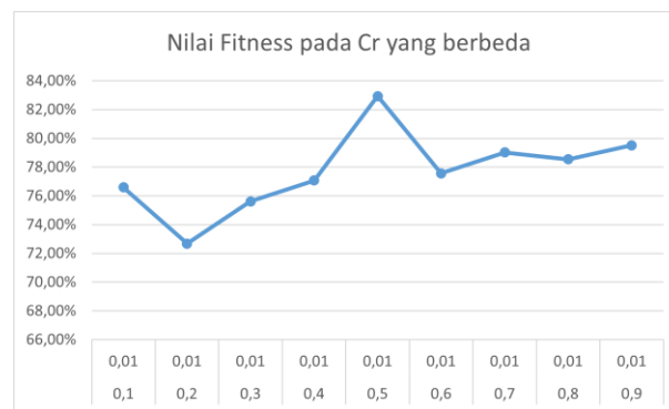
Gambar 7. Nilai Fitness dengan Cr yang berbeda
