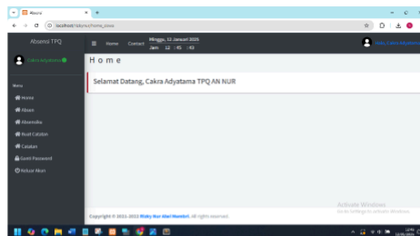
Gambar 14. Data Siswa
