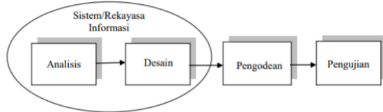
Gambar 2. Diagram Aktivitas
