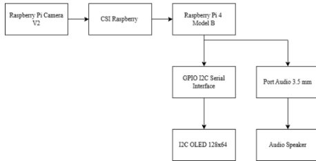
Gambar 1. Desain Perangkat Keras
