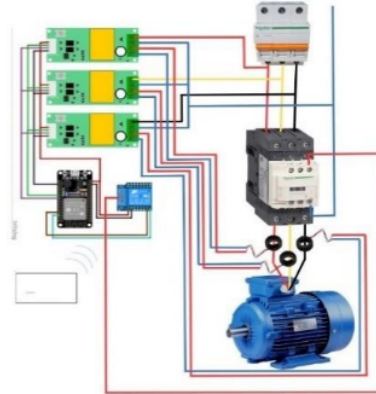
Gambar 3. Gambar rangkaian
