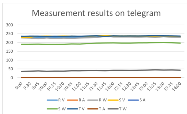
Gambar 8. Grafik Hasil pengukuran pada telegram
