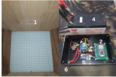
Gambar 11. Rangkaian Elektronika
