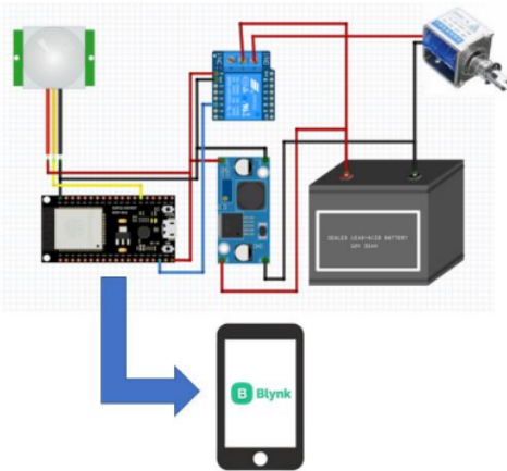
Gambar 8. Rancangan Perangkat Keras
