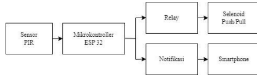
Gambar 2. Blok Diagram Sistem
