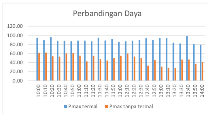
Gambar 7. Perbandingan PMAX termal dan tanpa termal
