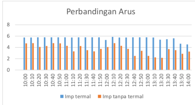
Gambar 8. Perbandingan IMP termal dan tanpa termal
