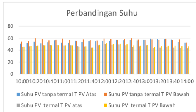
Gambar 9. Perbandingan Suhu termal dan tanpa termal
