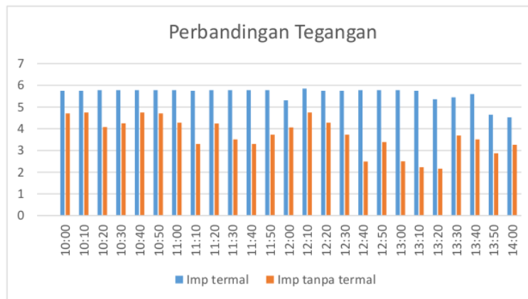
Gambar 6. Perbandingan VMP termal dan tanpa termal
