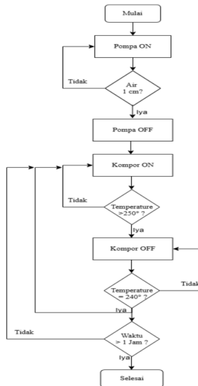
Gambar 2. Alur Sistem Proses Pemasakan Garam
