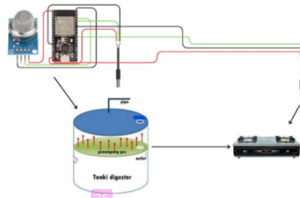
Gambar 5. Alur Pengambilan Data
