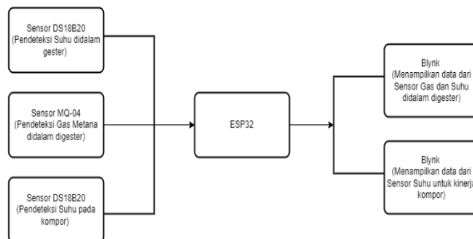
Gambar 1. Blok Diagram Sekarang
