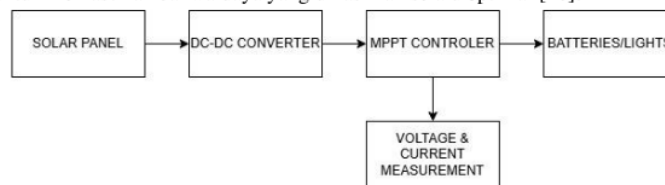
Gambar 1. Diagram blok MPPT
