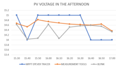
Gambar 16. PV Voltage di sore hari
