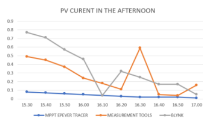
Gambar 17. PV Curent di Sore Hari
