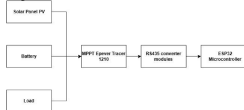
Gambar 2. Diagram desain alat
