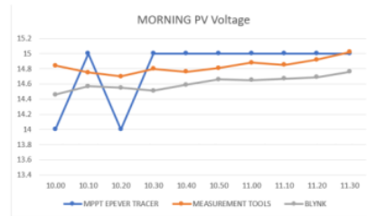
Gambar 10. Tegangan PV Pagi
