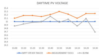
Gambar 13. Tegangan PV siang hari
