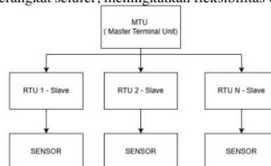
Gambar 3. Diagram blok yang menunjukkan aliran data
