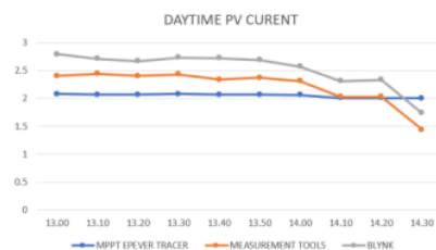
Gambar 14. PV Curent siang hari
