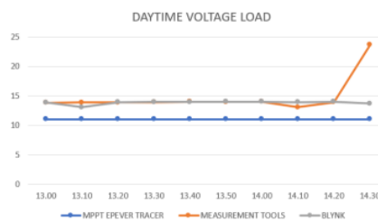
Gambar 15. Tegangan Beban Siang Hari
