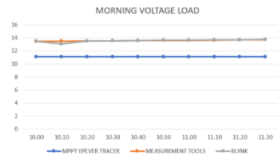
Gambar 12. Beban Pagi Voltage
