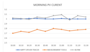
Gambar 11. PV Curent Pagi
