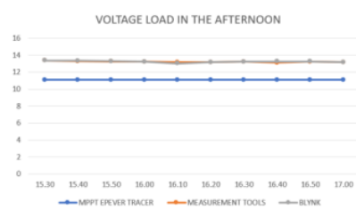
Gambar 18. Beban Tegangan di Sore Hari
