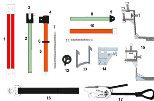
Gambar 1. Desain Teknik Konstruksi Alat Inovasi Triangle Support
