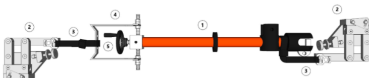
Gambar 4. Konfigurasi Kedua Alat Inovasi Triangle Support
