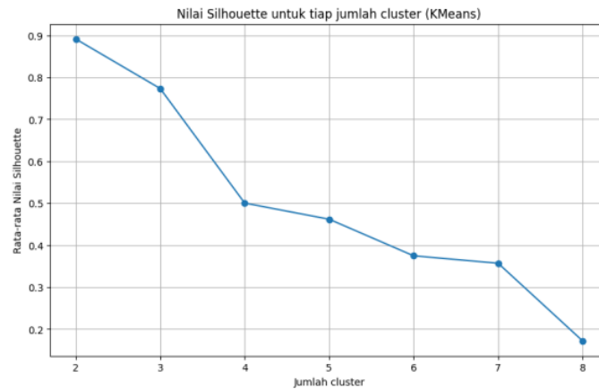
Gambar 4 Visualisasi Silhouette Score
