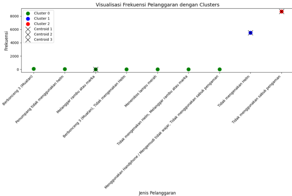
Gambar 3 Visualisasi Hasil Clustering
