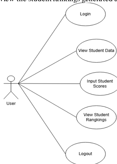
Fig. 3. Usecase Diagram
