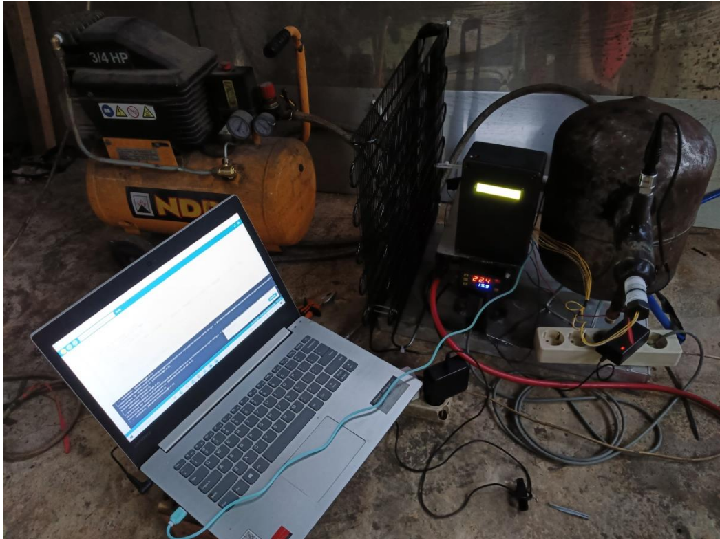
Gambar 5. Penempatan perangkat monitoring air dryer kompresor
