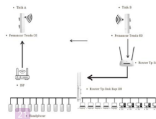
Gambar 2. Desain Jaringan
