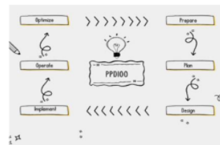
Gambar 1. Metode PPDIOO
