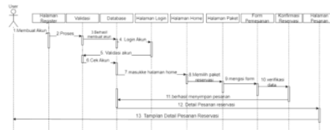
Gambar 4. Diagram Urutan untuk Proses Pemesanan
