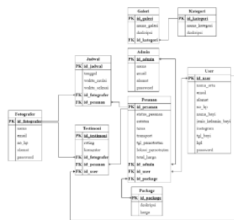
Gambar 5. Hubungan Antar Tabel
