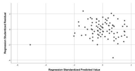
Gambar 2. Uji heterokedastisitas
