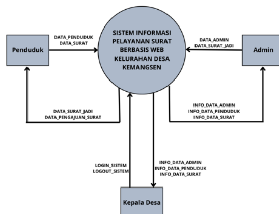
Gambar 2. Diagram Konteks
