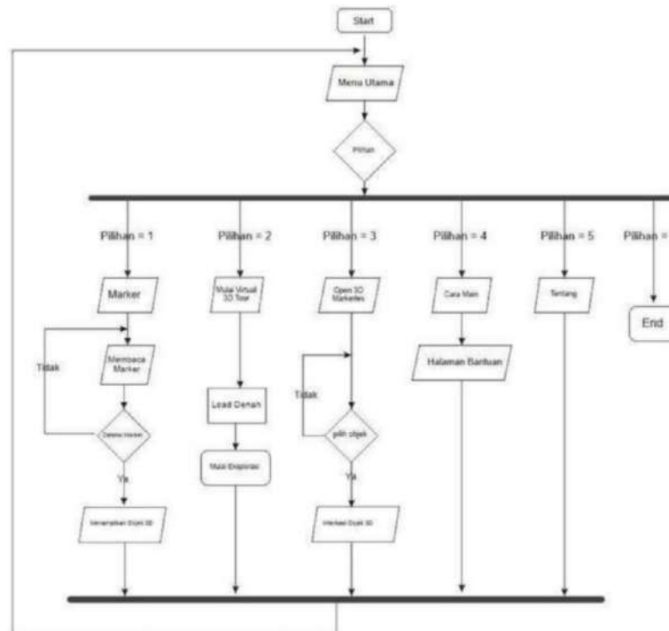
Gambar 3. Flowchart Aplikasi
