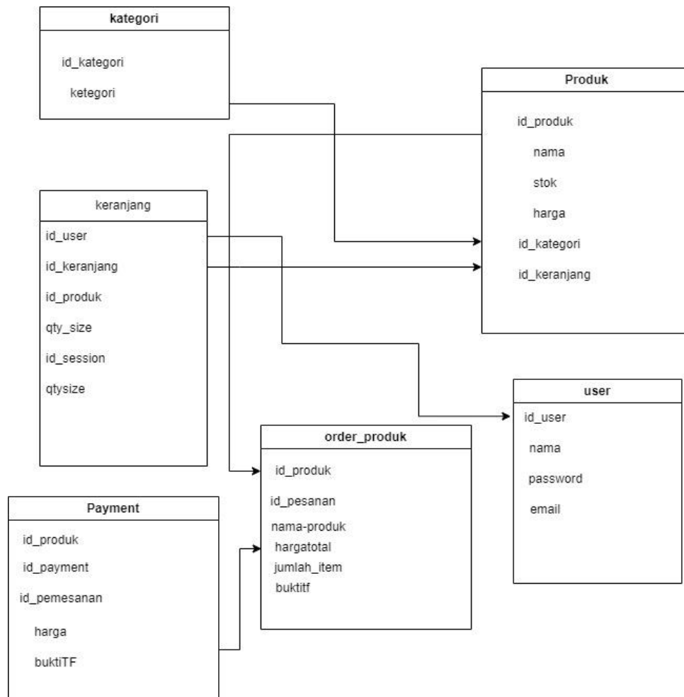
gambar 4, Relasi
