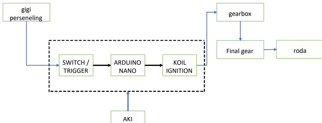
Gambar 3. Blok Diagram Pengoperasian Alat Dengan Alat Quicksifter [3]
