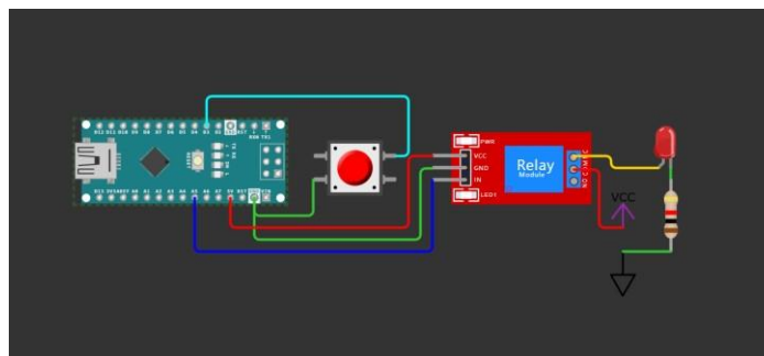
Gambar 7. Rangkaian Keseluruhan [7]
