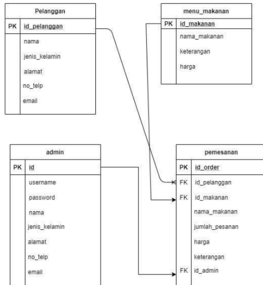
Gambar 6. Relasi Tabel
