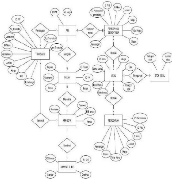
Gambar 5. ERD
