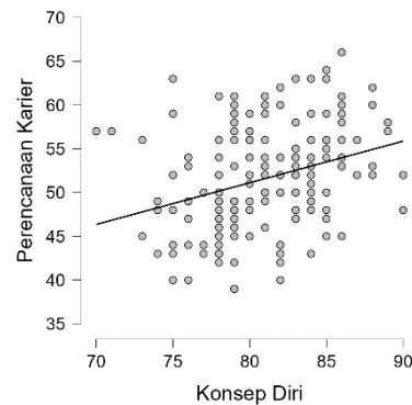
Grafik 1. Uji Linearitas
