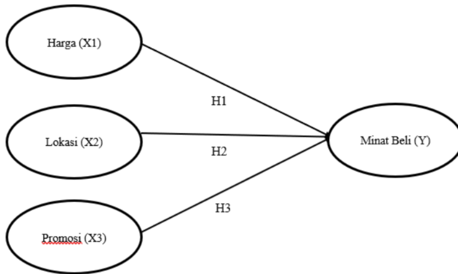
Gambar 1. Kerangka Konseptual
