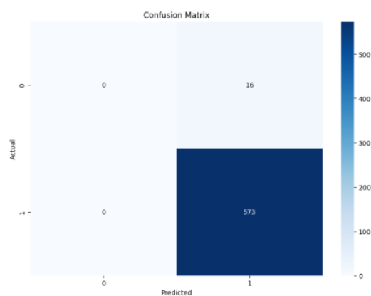
Gambar. 3. Hasil Visualisasi Confussion Matrix.
