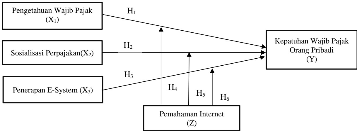
Gambar 1 : Kerangka Konseptual
