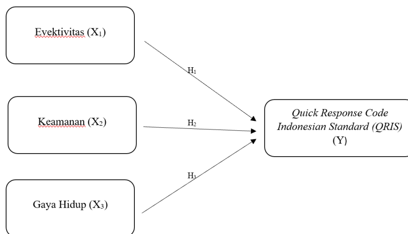
Gambar 1. Kerangka Konseptual
