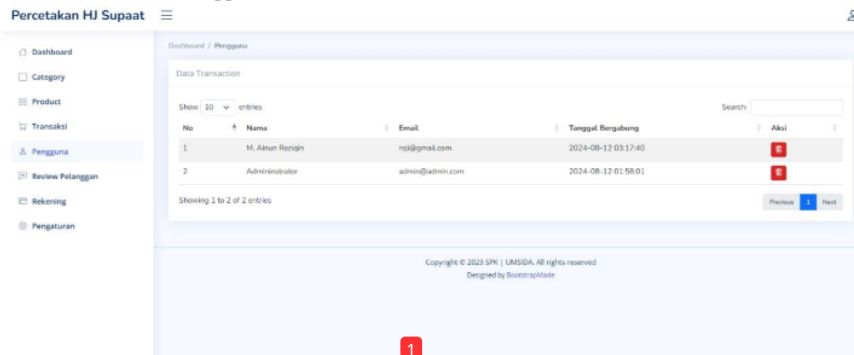
Gambar 3.9 Halaman Pengguna
