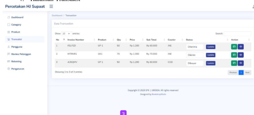
Gambar 3.8 Halaman Transaksi
