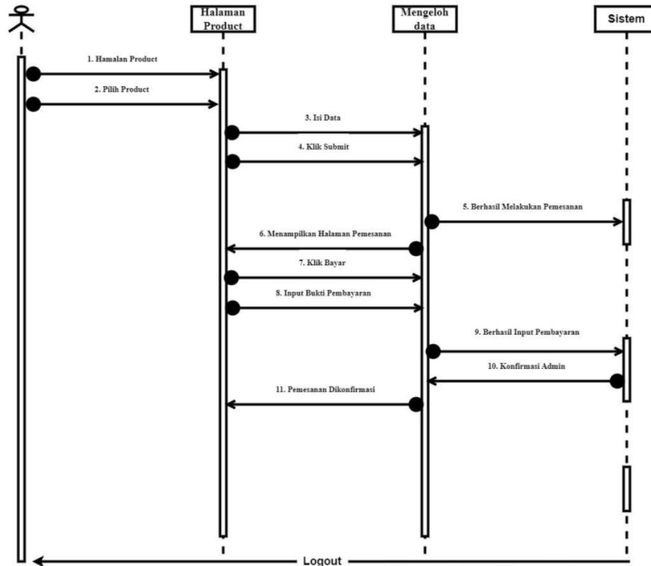
Gambar 3.4 Seq Pemesanan
