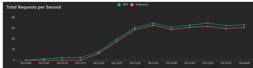
Gambar 3.21 Grafik RPS
