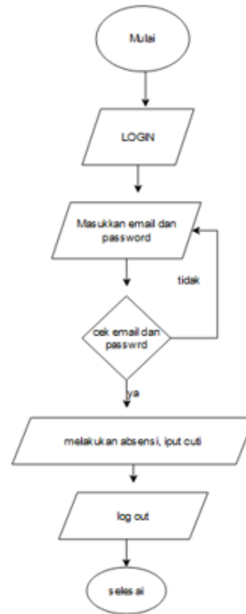
Gambar 3.2 Flowchart Karyawan
