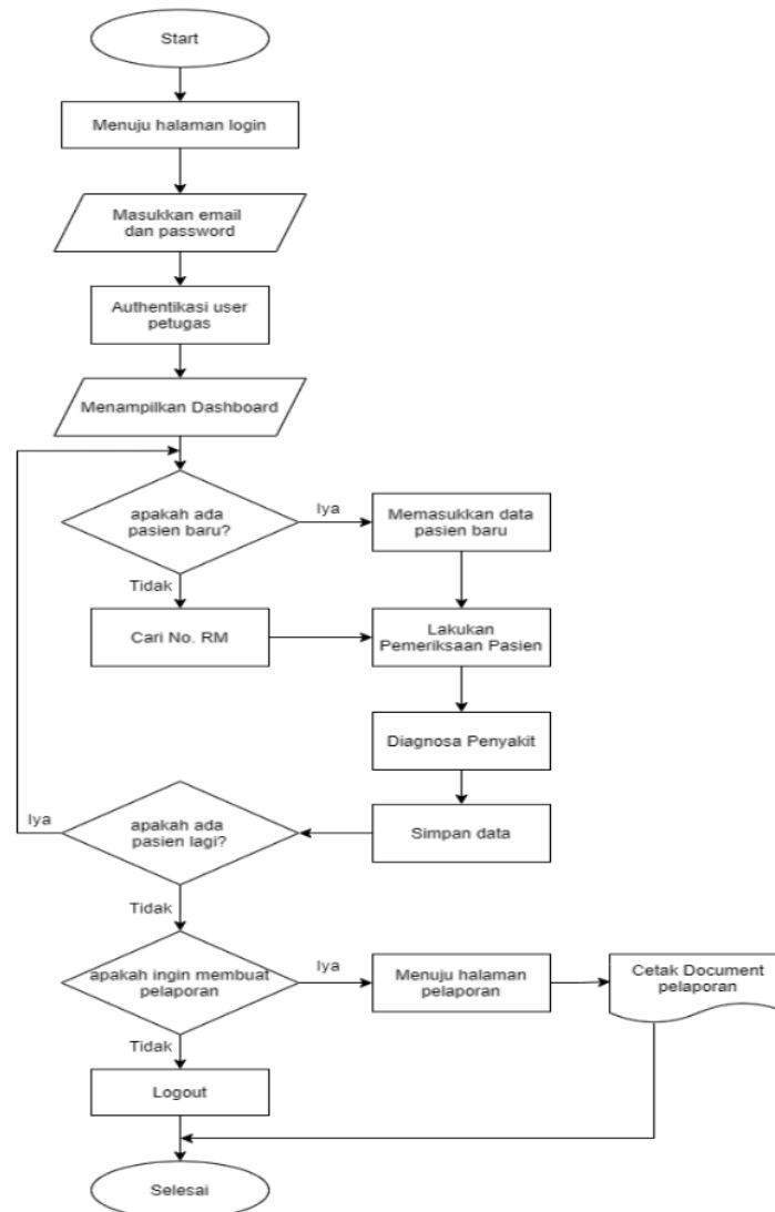
6 Gambar Error! No text of specified style in document..1 Flowchart Sistem Informasi Pendaftaran dan Pelaporan
