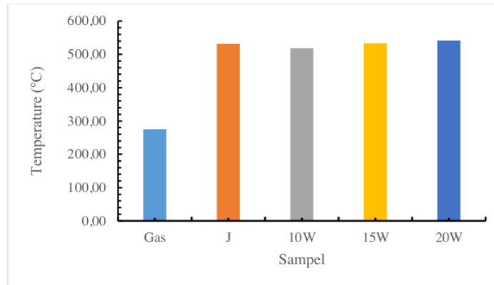
Gambar 3.8. Grafik Suhu Tertinggi BB
