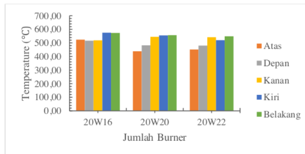
Gambar 3.7. Grafik Oli 20W - 40W
