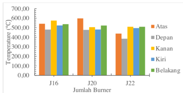
Gambar 3.4. Grafik Minyak Jelantah
