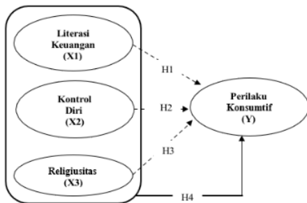
Gambar 1. Kerangka Konseptual
