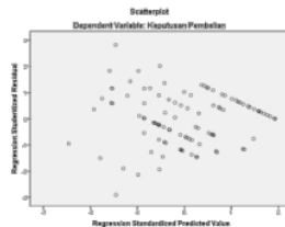
Gambar 2. Uji Heterokedastisitas
