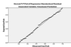
Gambar 1. Uji Normalitas
