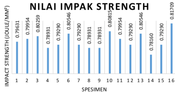
Gambar 18. Grafik nilai impact strength
