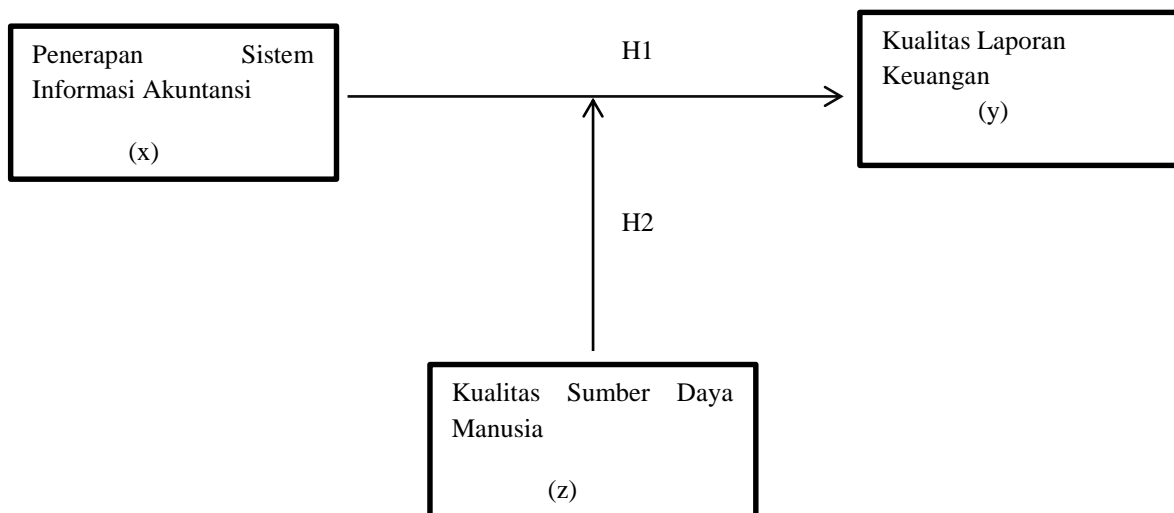
Gambar 1. Kerangka konseptual
