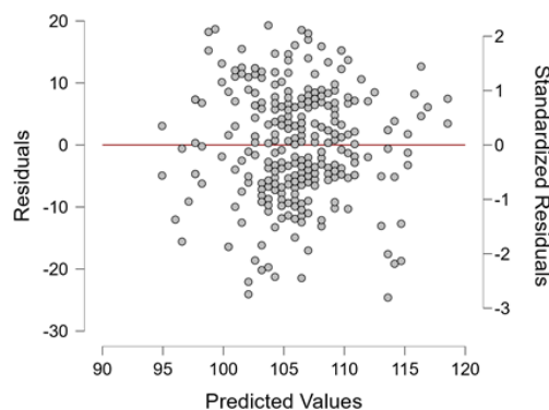
Gambar 2. Uji Linieritas
