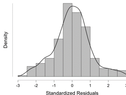
Gambar 1. Uji Normalitas
