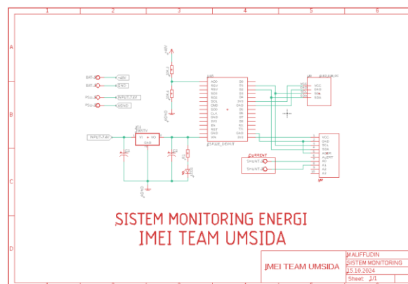
Gambar 4. Skema Rangkaian
