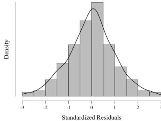
Gambar 1. Uji normalitas
