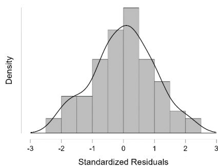
Gambar 1. Uji Normalitas
