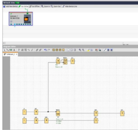
Gambar 5. Tampilan program Siemens LOGO dengan bahasa FBD
