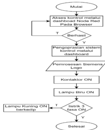
Gambar 1. Diagram alir sistem kontrol.
