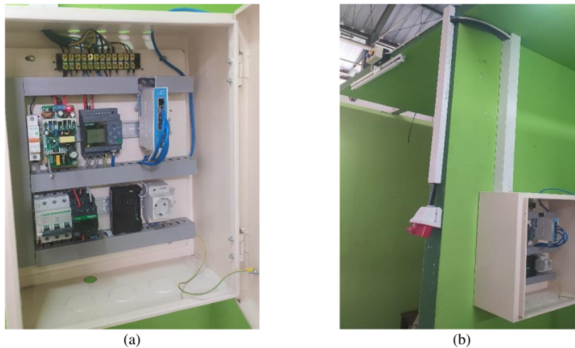
Gambar 4. (a) Hasil perancangan rangkaian elektrik; (b) hasil penempatan komponen.
