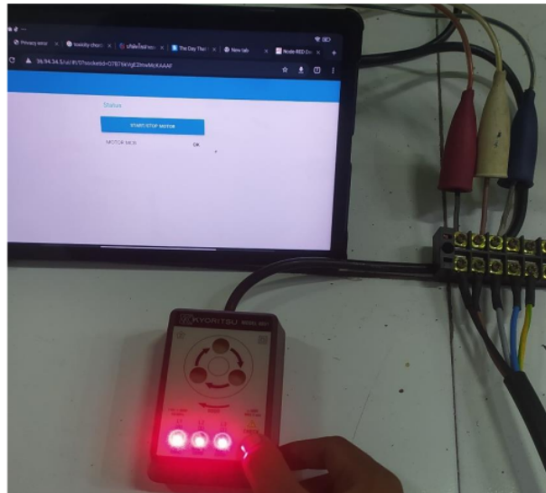
Gambar. 8 Pengujian urutan fasa.
