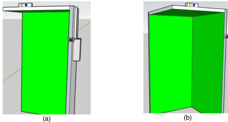
Gambar 3. (a) Penempatan komponen; (b) model bilik praktikum.
