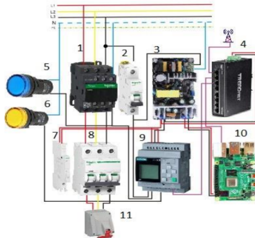
Gambar 2. Rangkaian elektrik.
