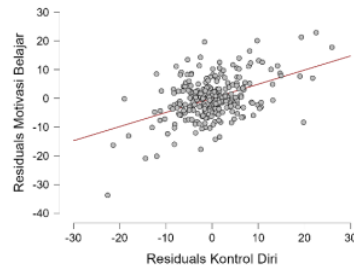
Gambar 3. Uji Linearitas Partial Regression Plots (Motivasi Belajar vs Kontrol Diri)
