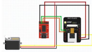
Gambar 4. Skema Rangkaian
