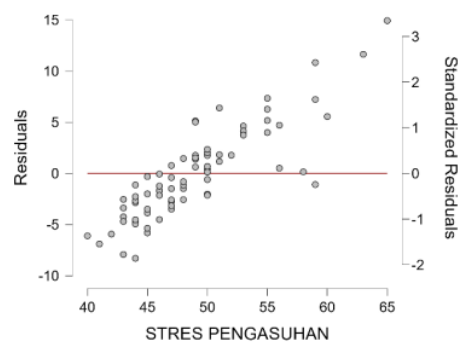
Gambar 1 : Uji Homoskedasitas
