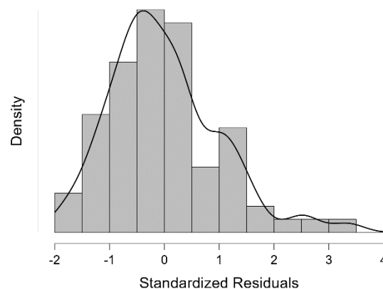
Gambar 1. Uji Normalitas dan Linieritas
