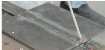
Gambar 7. Posisi Pengelasan 1G
