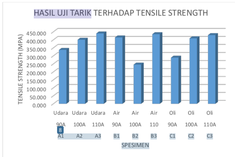
Gambar 20. Diagram Hasil Uji Tarik Spesimen terhadap Tensile Strength
