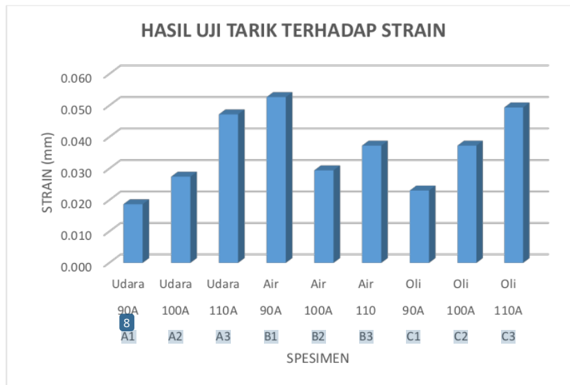
Gambar 21. Diagram Hasil Uji Tarik Spesimen terhadap Strain
