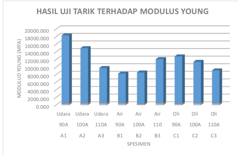
Gambar 22. Diagram Hasil Uji Tarik Spesimen Terhadap Moudulus Young
