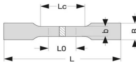
Gambar 8. Dimensi spesimen standar ASTM E8
