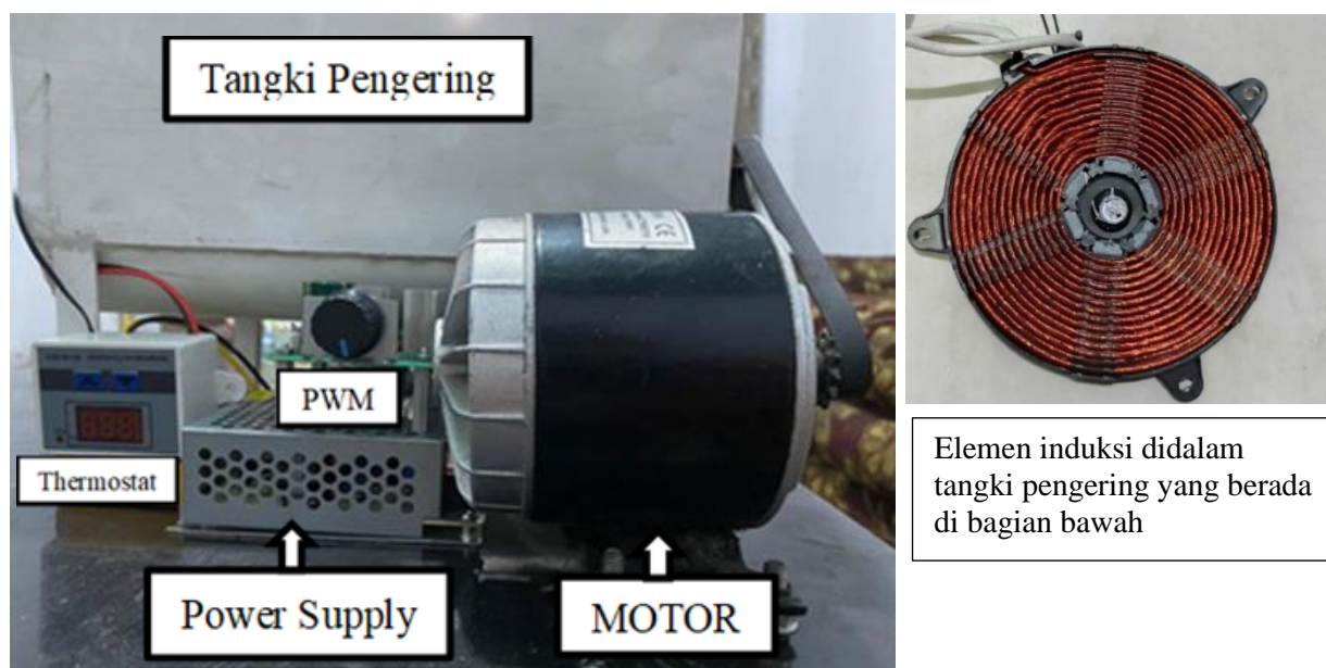
Gambar 4. Prototype Alat Sangrai Maggot BFS Menggunakan Induksi
